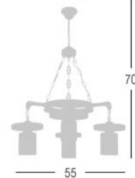
1715-4 SP 4 x E27 Max.60W
