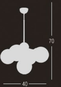
463-5 5xE14 Max.40W
