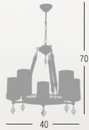
2016-5 KP-H 2016-5 SP- H 5xE27 Max.60W
