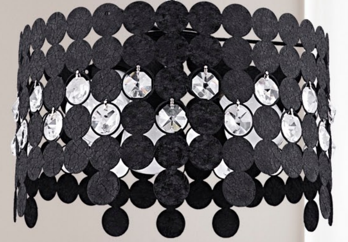
800-S h:60 Ø:32 / 3xE27 Max 40W 800-K h:60 Ø:60 / 3xE27 Max 40W 800-SK h:50 Ø:22 / 1xE27 Max 40W 800-PB h:50 Ø:22 / 1xE27 Max 40W
