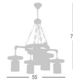
1715-5 GP 5 x E27 Max.60W
