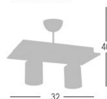
339-2 2 x E14 Max.40W
