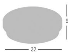
1040-2 2 x E27 Max.60W
